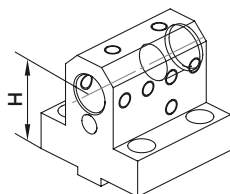
W1417 D25 - H=55 mm (Ø25 mm) W4437 D25 - H=75 mm (Ø25 mm)
