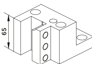
Z2413 - 25x25 mm
