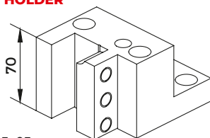
W2413 - 25x25 mm
