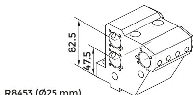
R8453 (Ø25 mm)
