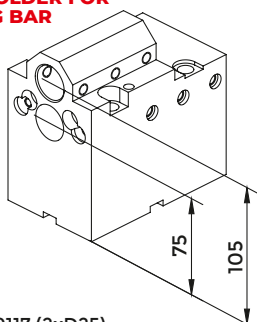
KMS-T10117 (2xD25)
